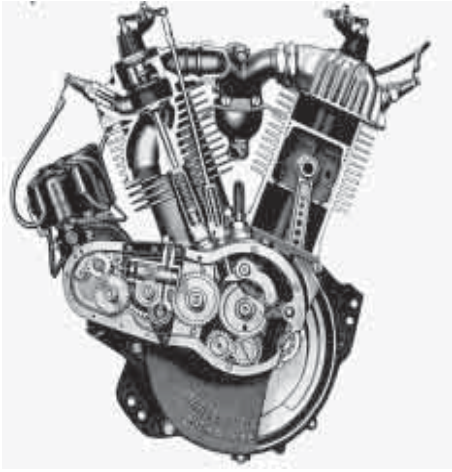
Motor der Typen J und F
