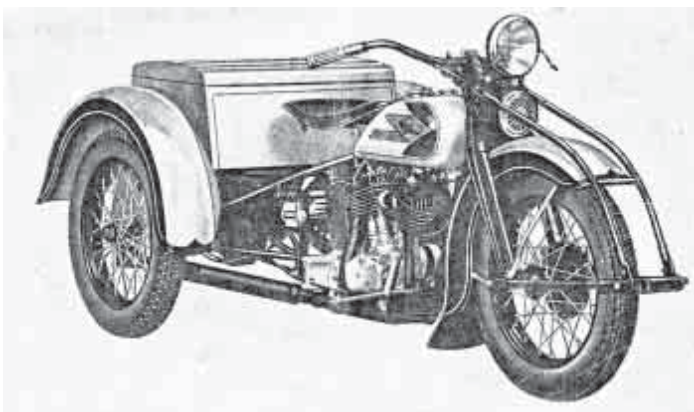
35 G 750-er Servi-Car (mit kleiner Box)
