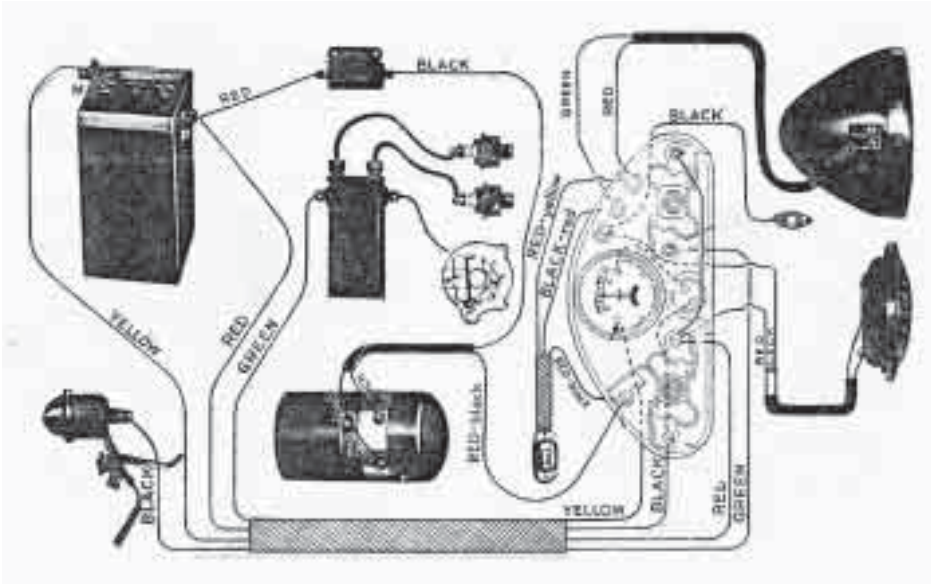
Elektrische Anlage
